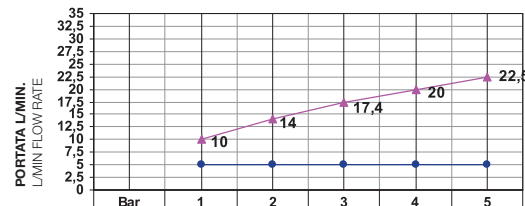
USCITA DOCCETTA / HANDSHOWER EXIT
