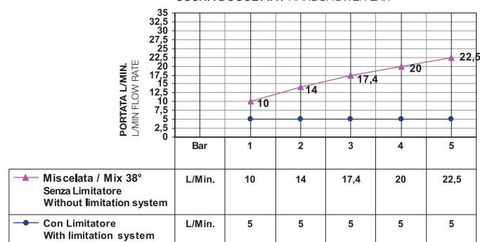
USCITA DOCCETTA / HANDSHOWER EXIT
