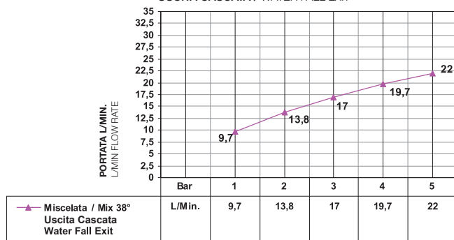
USCITA CASCATA / WATER FALL EXIT
