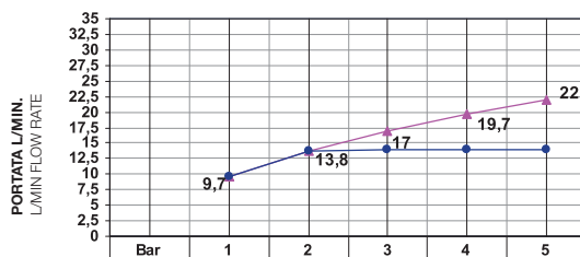
USCITA SOFFIONE / SHOWER HEAD EXIT
