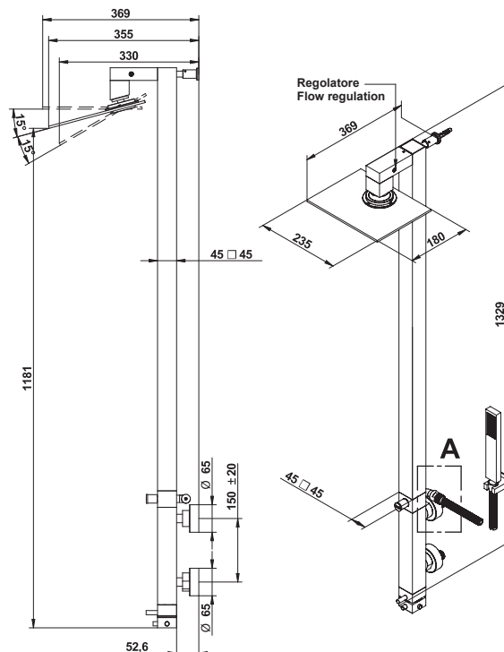
DETTAGLIO / DETAIL A
