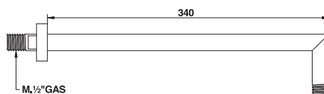
CODICE/CODE 805 BRACCIO DOCCIA MM 340 IN OTTONE. 340 MMS BRASS SHOWER ARM.
