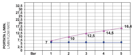
USCITA DOCCIA / SHOWER EXIT
