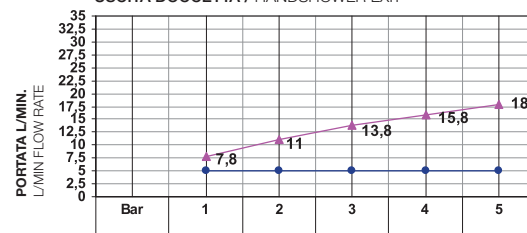
USCITA DOCCETTA / HANDSHOWER EXIT
